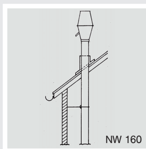
EXA ® -Dachausblas-Set
