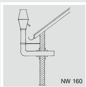
EXA ® -Wandausblas-Set
